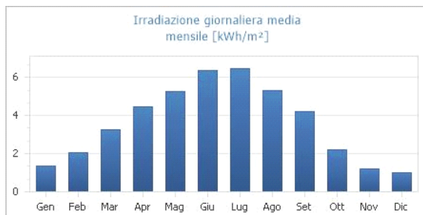
Irradiazione giornaliera media mensile sul piano orizzontale [kWh/m 2 ] - Fonte dei dati: UNI 10349:2016 - Stazione di rilevazione: Milano - via Juvara
